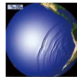
2011年チリ地震津波の伝播の様子
